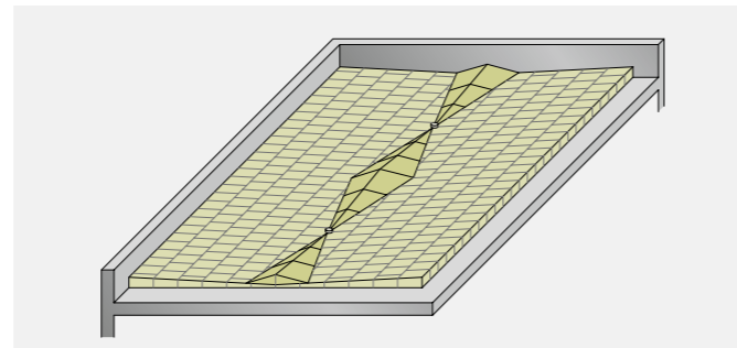
Systemskizze des Gefälledachsystems Georock mit Punktentwässerung Ke Brock
